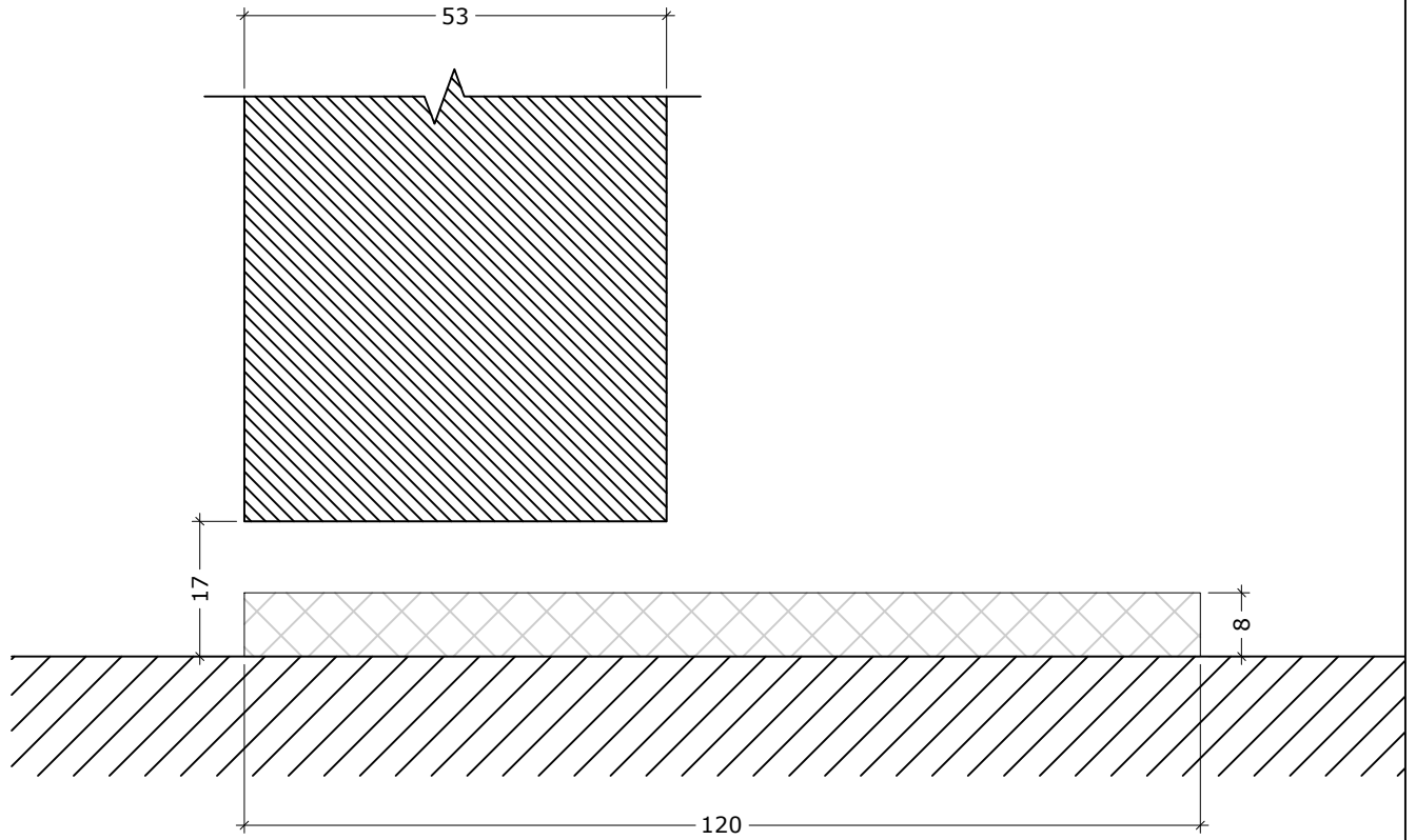
DEKO PD detail (Portal door)
