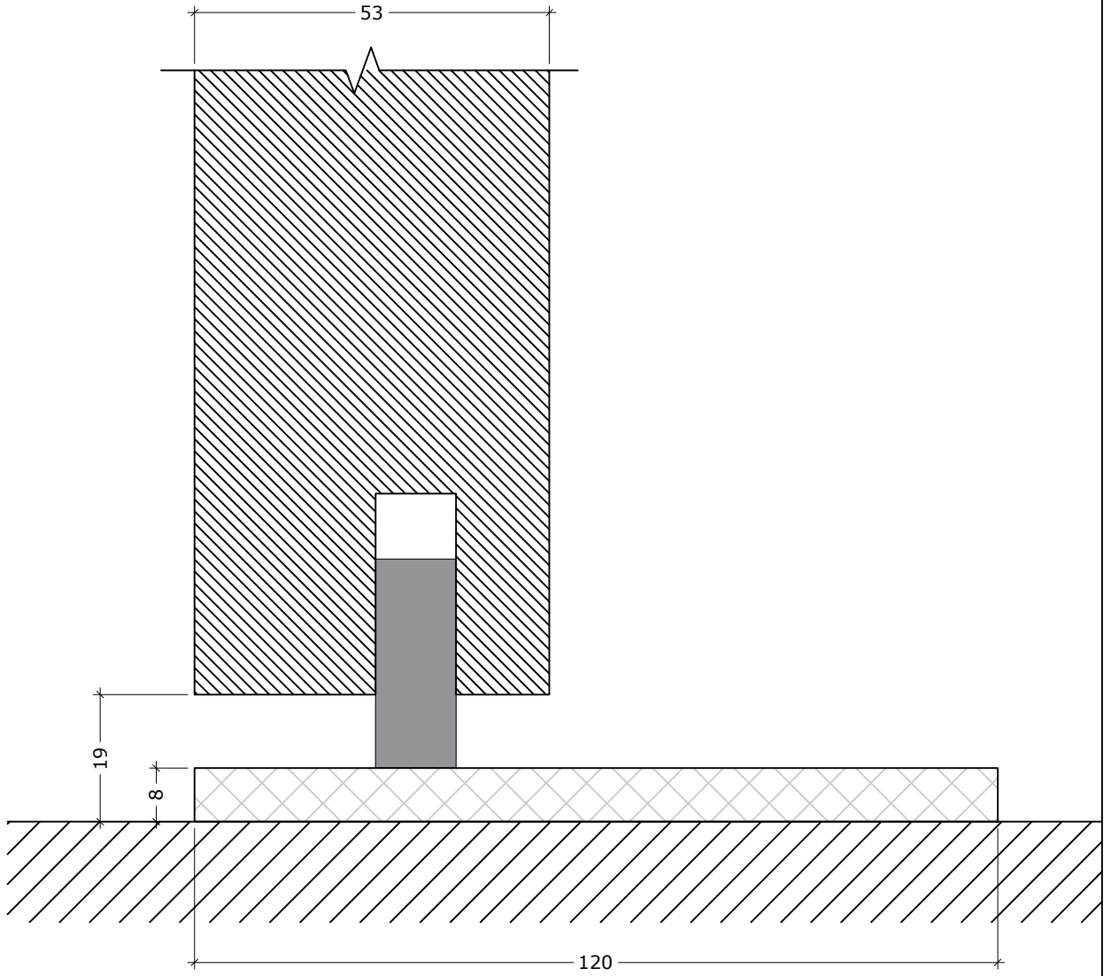
DEKO PD detail (Portal door)
