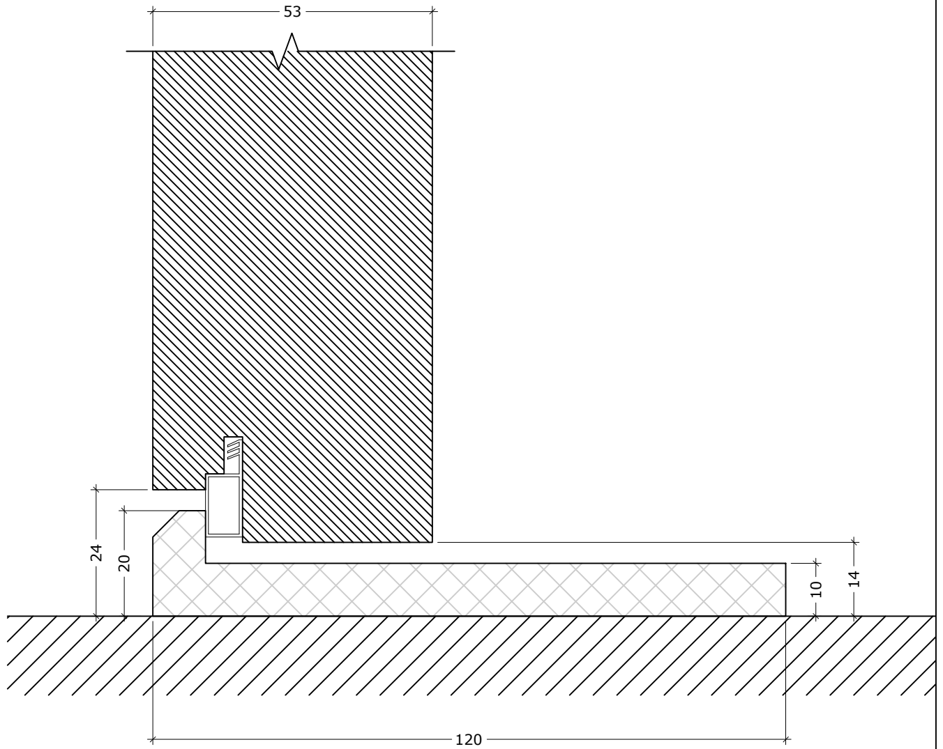
DEKO PD detail (Portal door)
