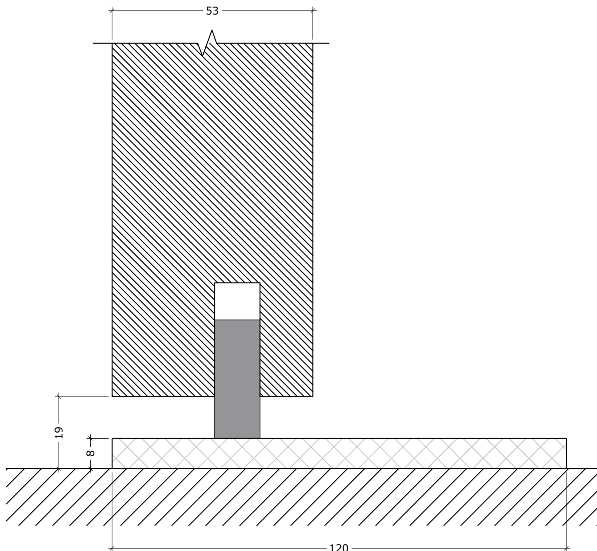
DEKO PD detail (Portal door)
