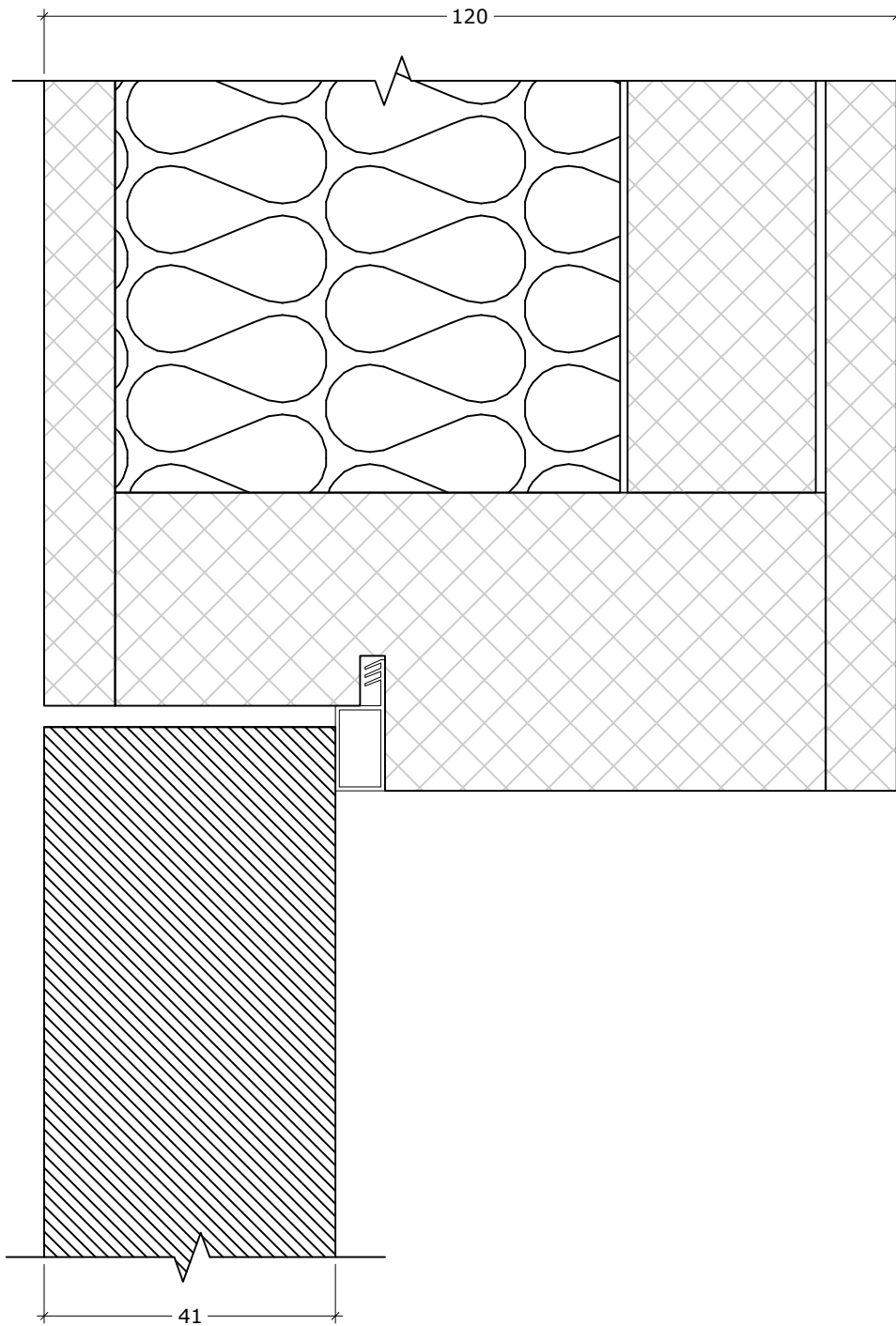
DEKO PD detail (Portal door)
