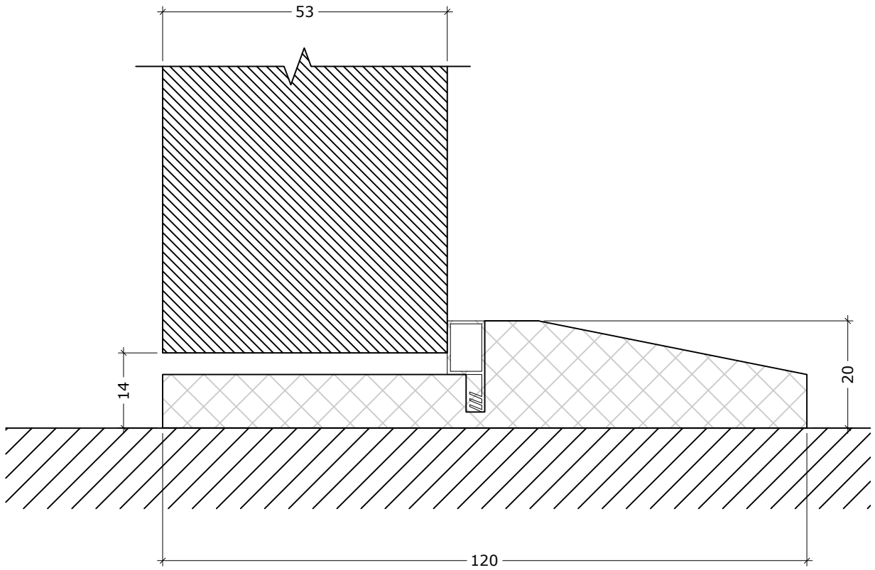
DEKO PD detail (Portal door)
