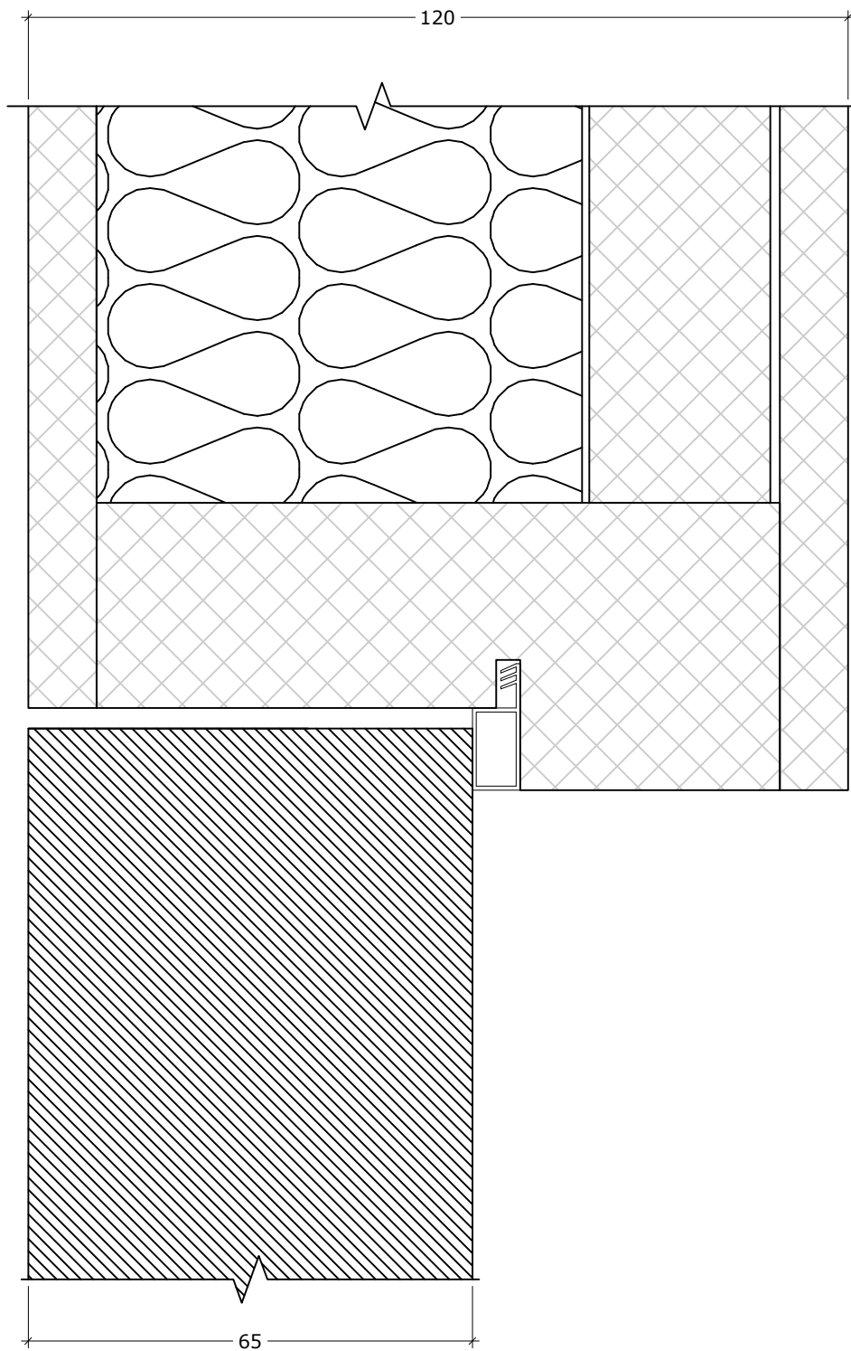
DEKO PD detail (Portal door)
